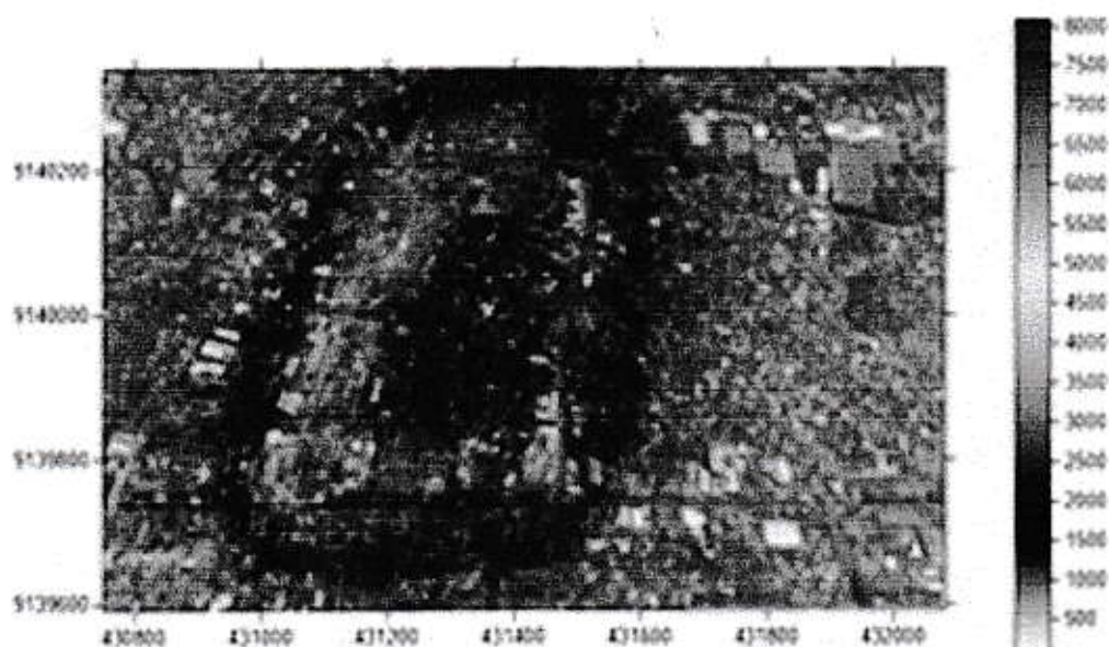
Simulasi pencemaran CO di Yogyakarta
